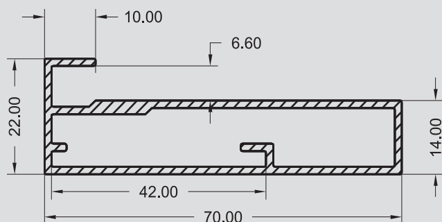
SP - 0281 0,761 KG/M
