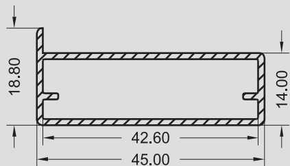
SP - 0218 0,387 KG/M
