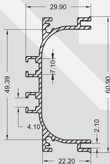
SP - 0285 0,601 KG/M
