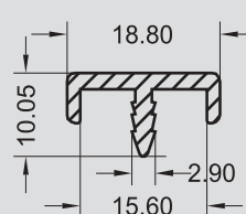
SP - 0023/A 0,181 KG/M
