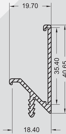
SP - 0289 0,337 KG/M
