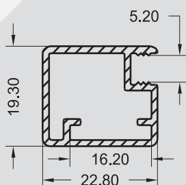
SP - 0043 0,321 KG/M
