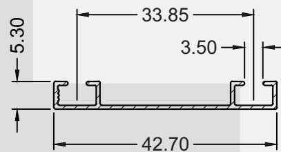
SP-0049/LL 0,139 KG/M
