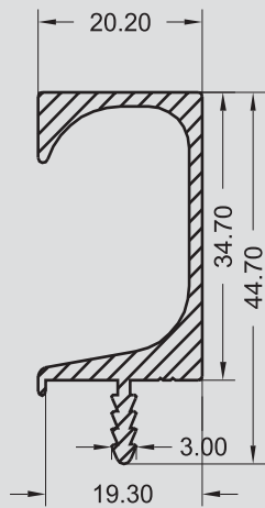
SP - 0021 0,498 KG/M
