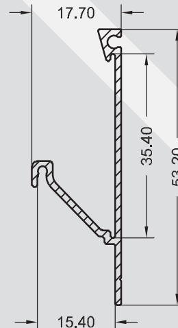
SP - 0456 0,289 KG/M
