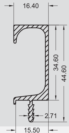
SP - 0080 0,364 KG/M
