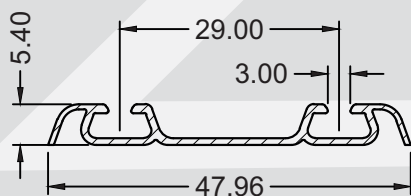
SP - 0282 0,193 KG/M
