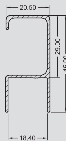
SP - 0142 0,348 KG/M
