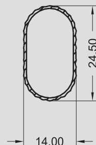
TUB - 0001/ASL 0,107 KG/M
