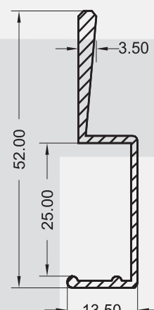
SP - 1815 0,337 KG/M
