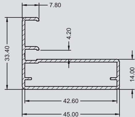
SP-0088 0,529 kg/m
