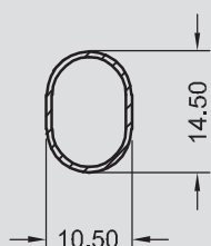
TUB - 0001 0,184 KG/M
