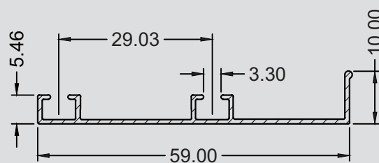
SP - 0381 0,213 KG/M
