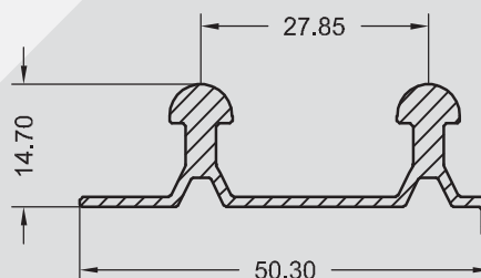
SP - 1322 0,474 KG/M
