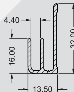
SP - 0007 0,279 KG/M
