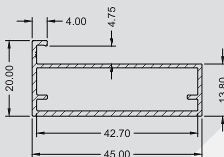
SP-2163 0,410 kg/m
