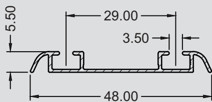
SP - 0014 0,178 KG/M
