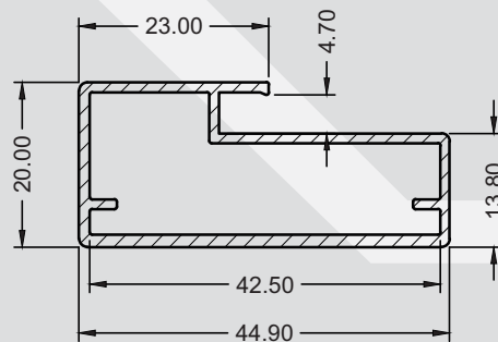
SP-0055 0,482 kg/m
