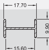
SP - 0089/LL 0,097 KG/M
