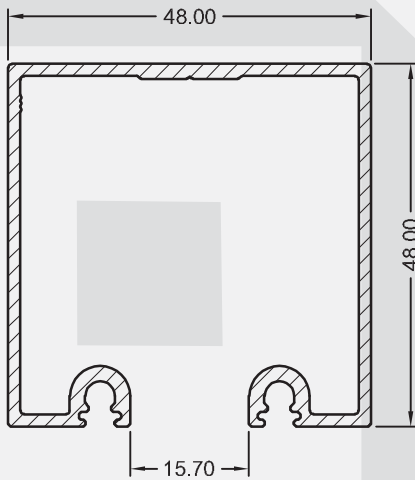
SP-4848/L 0,866 KG/M
