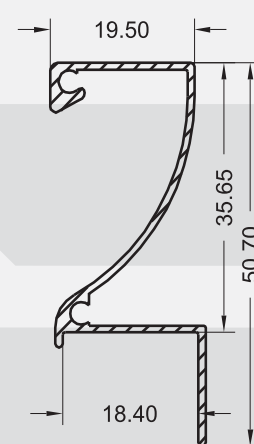
SP - 0309 0,288 KG/M
