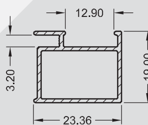
SP - 0484 0,238 KG/M
