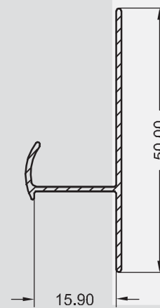
SP - 0307 0,203 KG/M
