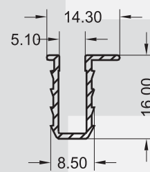
SP - 0067 0,134 KG/M
