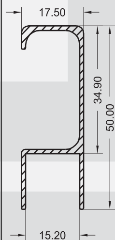
SP - 0153 0,330 KG/M
