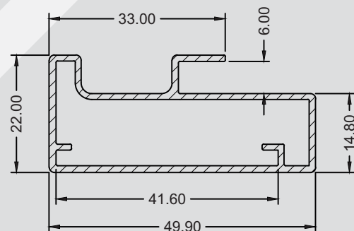
SP-0072 0,532 kg/m
