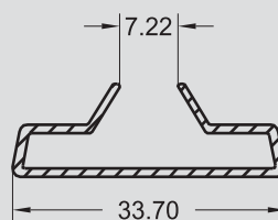
SP - 0024 0,194 KG/M
