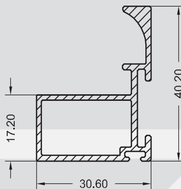
SP - 0339 0,545 KG/M
