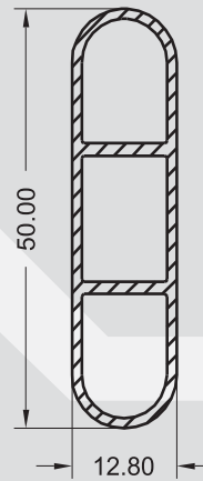
SP - 0361 0,509 KG/M
