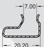
SP - 0016 0,095 KG/M
