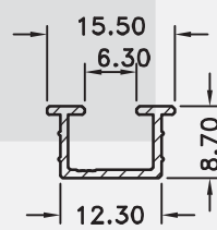
SP - 0141 0,095 KG/M
