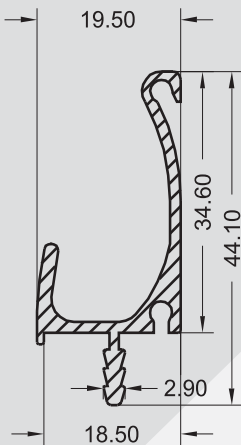
SP - 0148 0,372 KG/M
