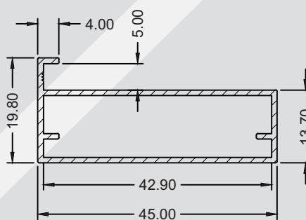
SP-2163/L 0,352 kg/m
