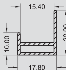
SP - 0062/R 0,195 KG/M
