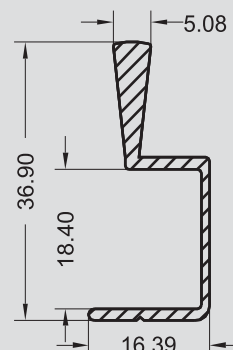
SP - 0098 0,314 KG/M
