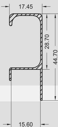
SP - 0243 0,246 KG/M
