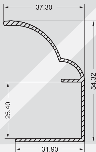
SP - 0792 0,435 KG/M
