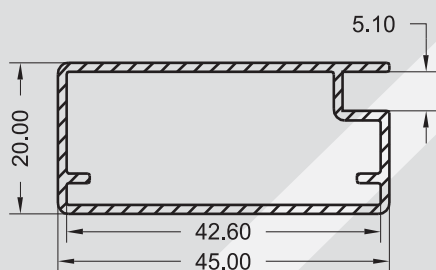
SP - 0026 0,447 KG/M
