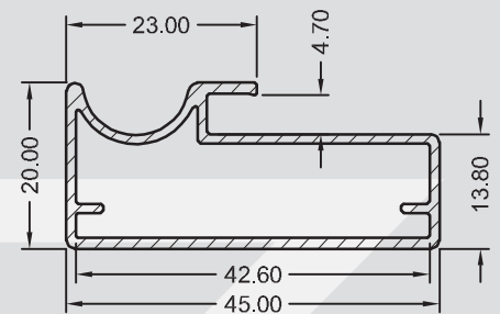
SP - 0051 0,466 KG/M
