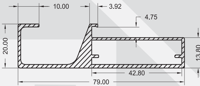
SP - 0075 0,867 KG/M
