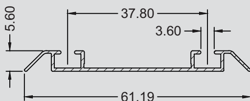
SP - 1847 0,207 KG/M
