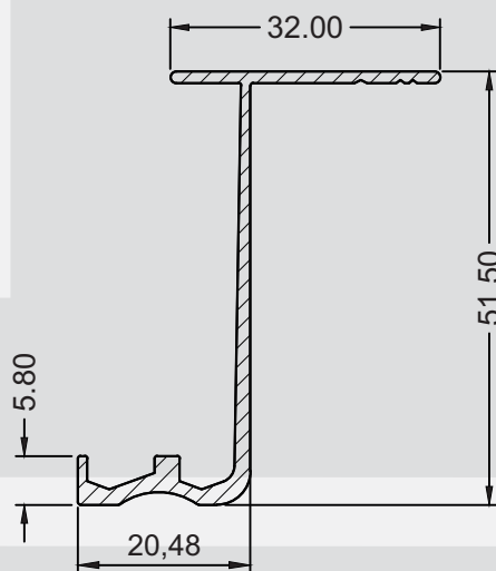
SP - 0008 0,458 KG/M
