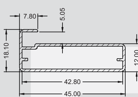
SP-0272 0,380 kg/m
