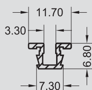
SP - 0018 0,077 KG/M
