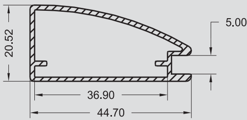
SP - 0010/A 0,401 KG/M
