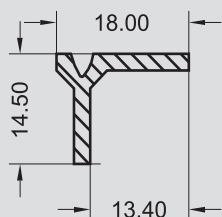
SP - 0038 0,160 KG/M
