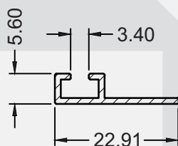
SP - 0210 0,105 KG/M
