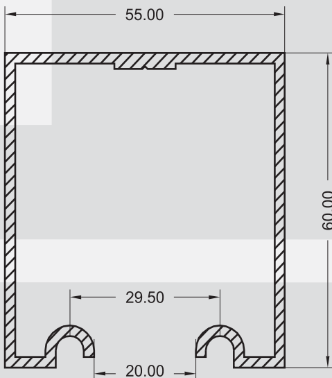
U - 1048 1,200 KG/M
