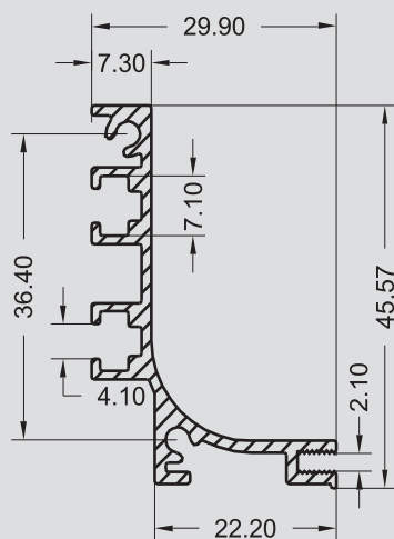
SP - 0284 0,453 KG/M
