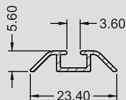
SP - 1848 0,106 KG/M
